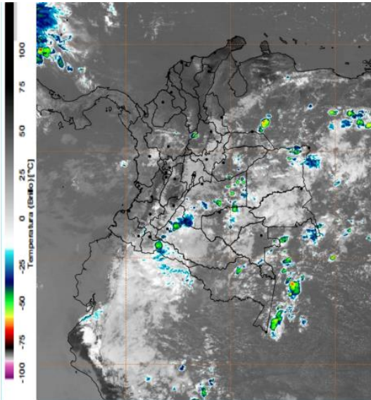
Imagen GOES East Canal Infrarrojo, 15 de julio de 2020. Hora 11:50 HLC. Fuente: IDEAM-GOES 167
