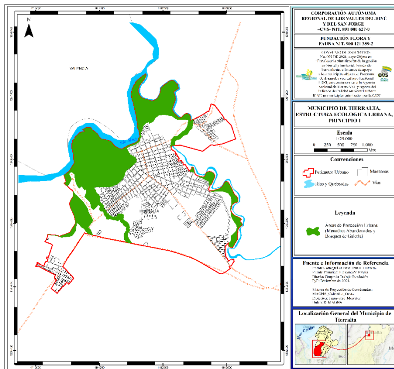
Mapa 8: Áreas de importancia ambiental urbanas.
