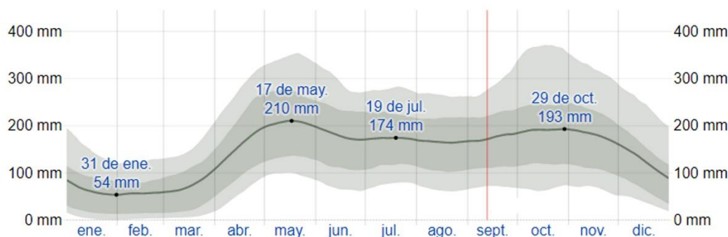
Ilustración 1: Precipitación mensual promedio
