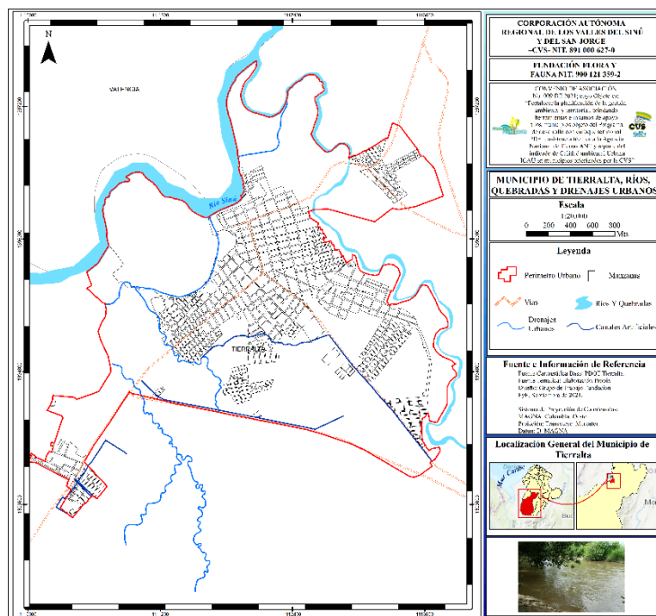
Mapa 7: Hidrología área urbana Municipio de Tierralta
