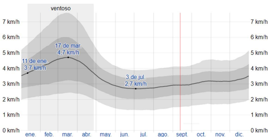
Ilustración 5: Velocidad promedio del viento
