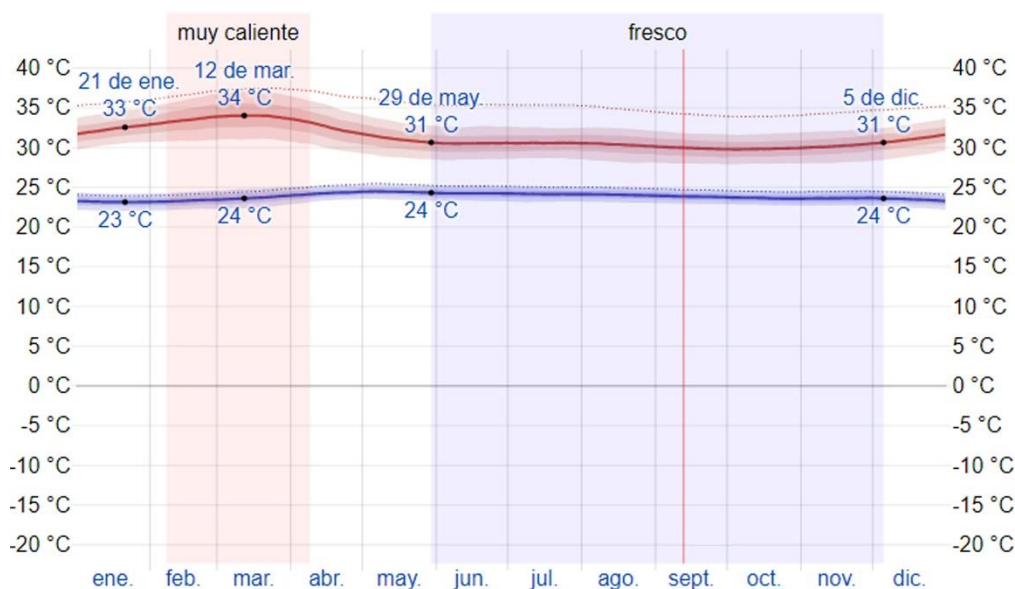
Ilustración 2: Temperatura máxima y mínima promedio
