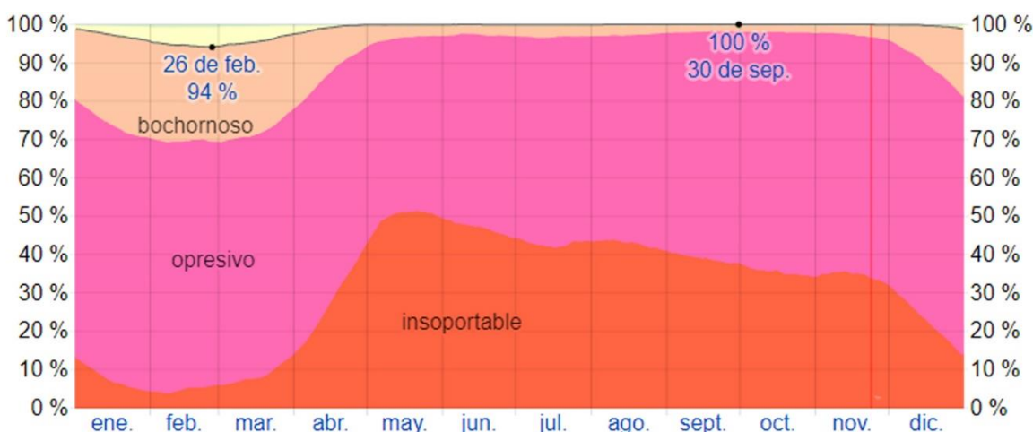
Ilustración 3: Humedad relativa
