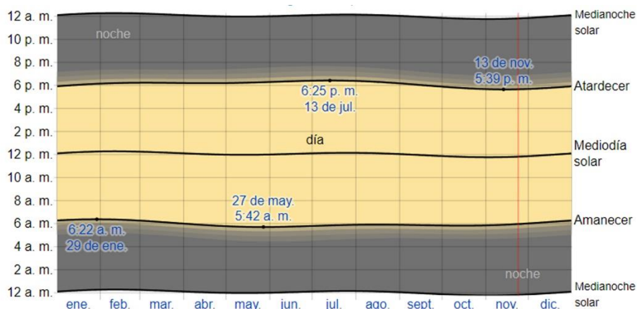
Ilustración 4: Período solar
