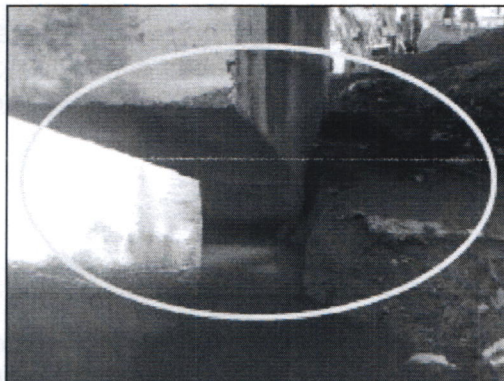
Imagen 3 y 4. Cauce del caño Aguas Prietas y estribo norte dentro del cauce del Caño Aguas Prietas disminuyendo la sección hidráulica, borde libre de aproximadamente 1m.
