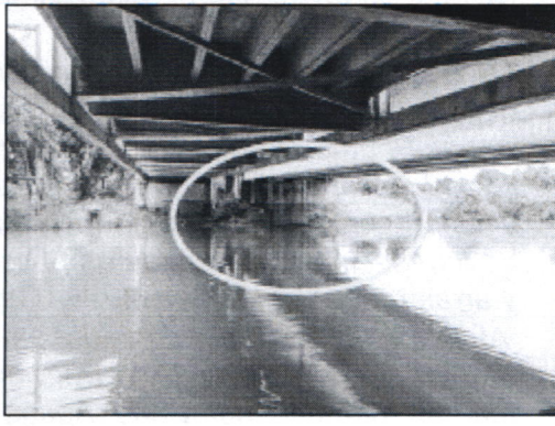
Imagen 5 y 6. Estribo sur dentro del cauce del Caño Aguas Prietas disminuyendo su sección hidráulica.
