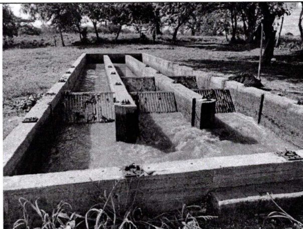
Residuos y lodos dispuestos a los lados de la estructura de tratamiento preliminar
